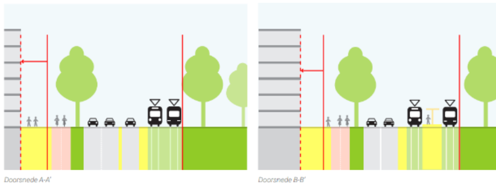
Figuur 2-23 Voorbeeldprofiel Maanweg
