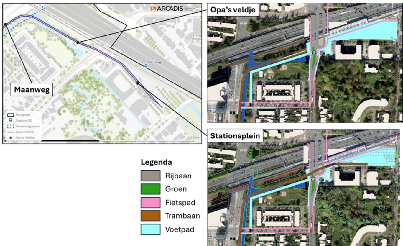
Figuur 2-33 De twee ontwerpen voor de eindhalte van de Vlietlijn in Voorburg
