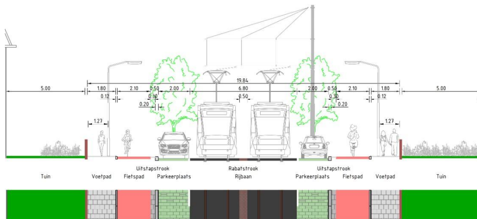
Figuur 2-28 Voorbeeld uitwerking Prinses Mariannelaan (west)
